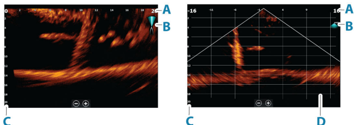
LiveSight-näkymä eteenpäin
